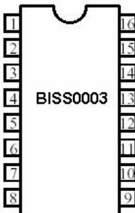
引脚说明
