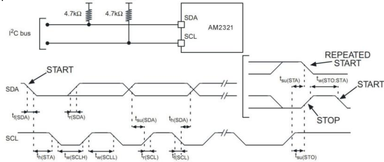
图 13: AM2321 典型的 I2C 总线应用电路和时序图
