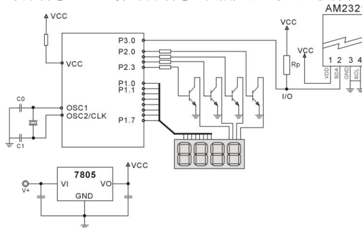
图 19： AM2321 单总线典型电路
