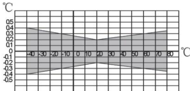
温度误差图
