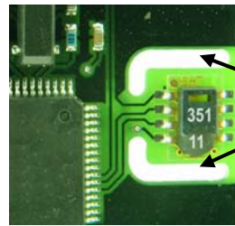
图 13 SHT1x PCB 安装举例
