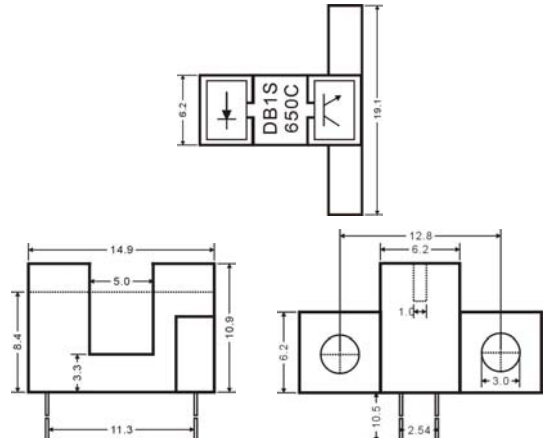
图.6 外形尺寸图 (单位: 毫米 ±0.1)
