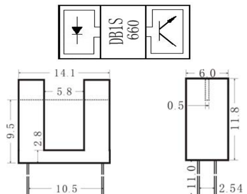
图.6 外形尺寸图 (单位: 毫米 ±0.1)
