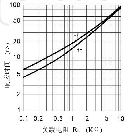
图.4 响应时间与负载电阻
