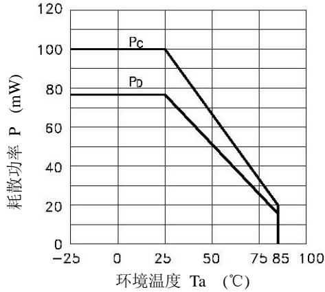
图.1 耗散功率与环境温度
