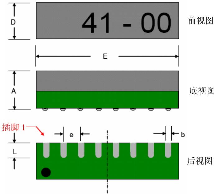
封装图 HMC1041Z (8 插脚 LPCC, 尺寸单位: mm)
