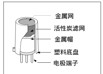
图1b. 标准形状
