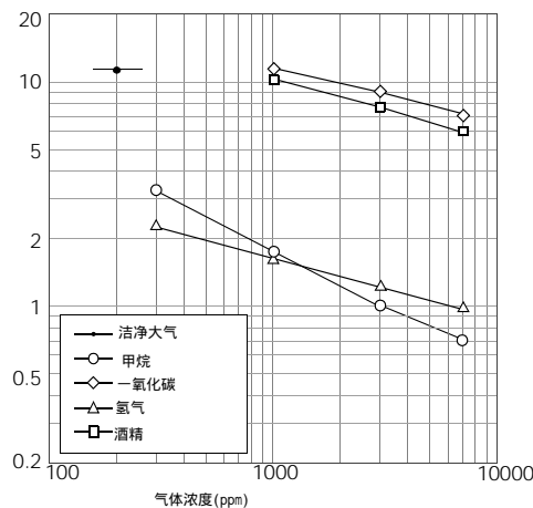
图3. 甲烷在高温时候的气体感度特性
