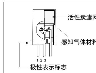
图1c. 电极端子配置
