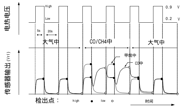
图2. SB-95-12的电热驱动条件和传感器输出变化
