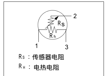
图1d. 等价电路
