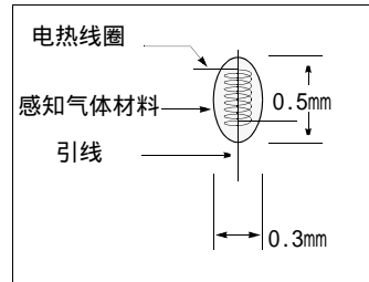
图1a. 感知气体素子
