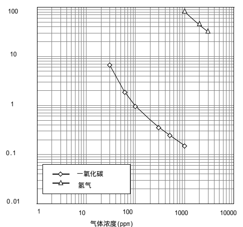
图4. 一氧化碳在低温时的感度特性
