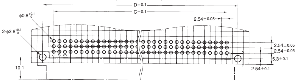
印刷基板加工尺寸 (BOTTOM VIEW)
