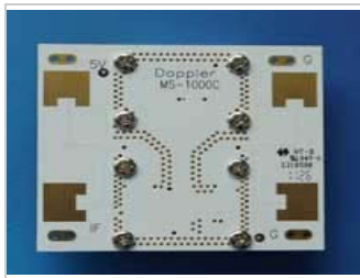
SMW-1000C微波传感器
