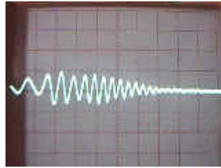
虑波处理后的 3.33M 信号回波 图 27
