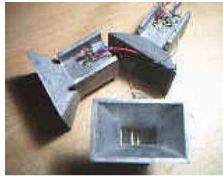
微波波导腔体振荡器 微波雷达测距传感器 06
