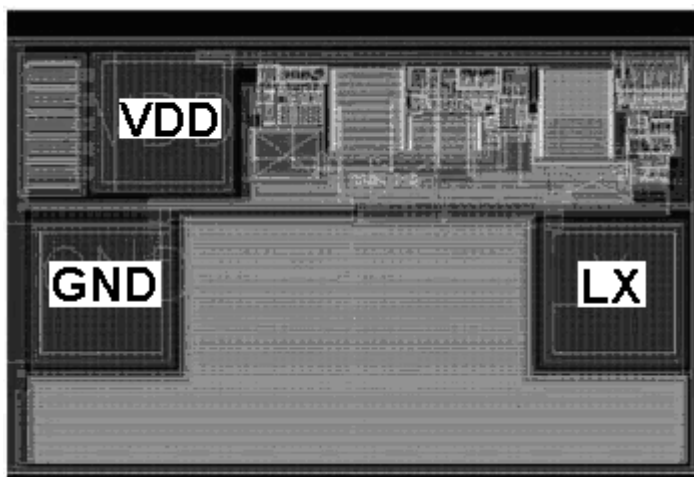
PAD 脚位图 (IC 衬底接 GND)
