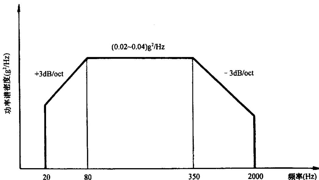
图 1 随机振动功率谱密度
