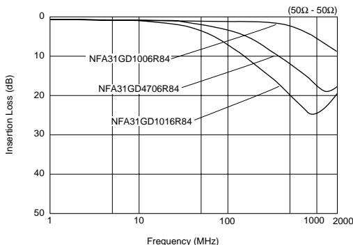
Insertion Loss(Typ.)
