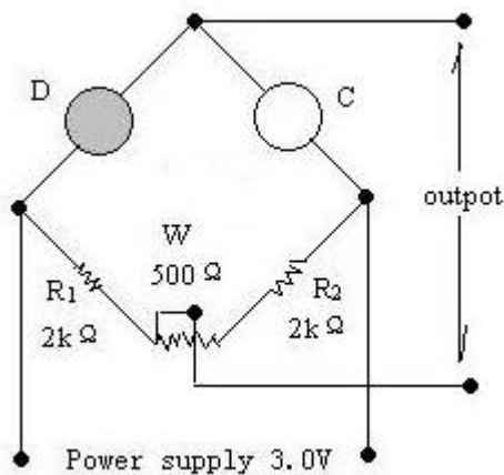
基本测试电路
