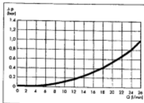
压力损失图
