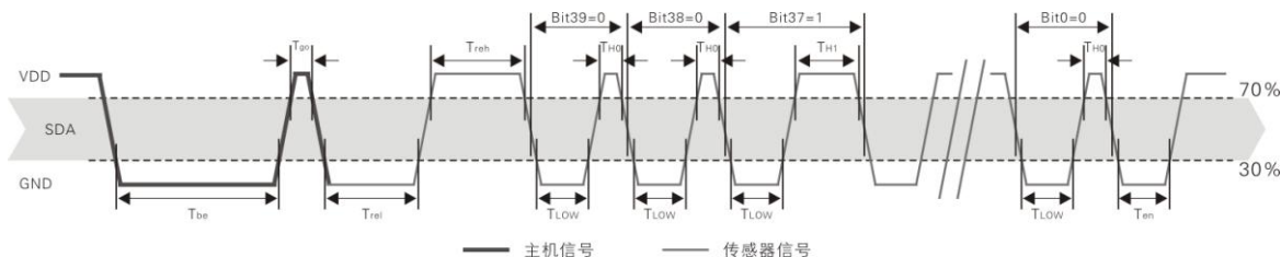
图 6: AM2303 单总线通信时序
