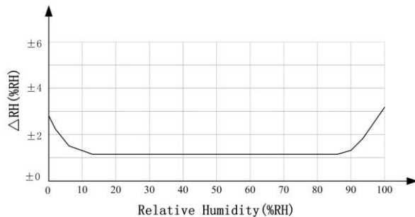
图 2: 25°C时 AM2303 的相对湿度最大误差
