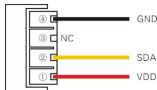
图 1： AM2303 引脚分配图
