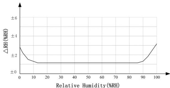
图 2: 25°C时 AM2305 的相对湿度最大误差
