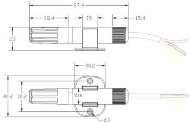
外形尺寸（单位：mm）
