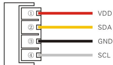
图 1: AM2315 接线图
