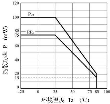
图.1 耗散功率与环境温度
