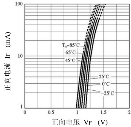
图.2 正向电流与正向电压
