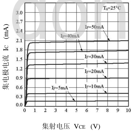
图.3 集电极电流与集射电压
