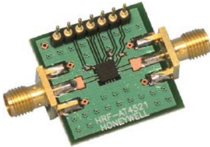
HRF-AT4521 评估板
