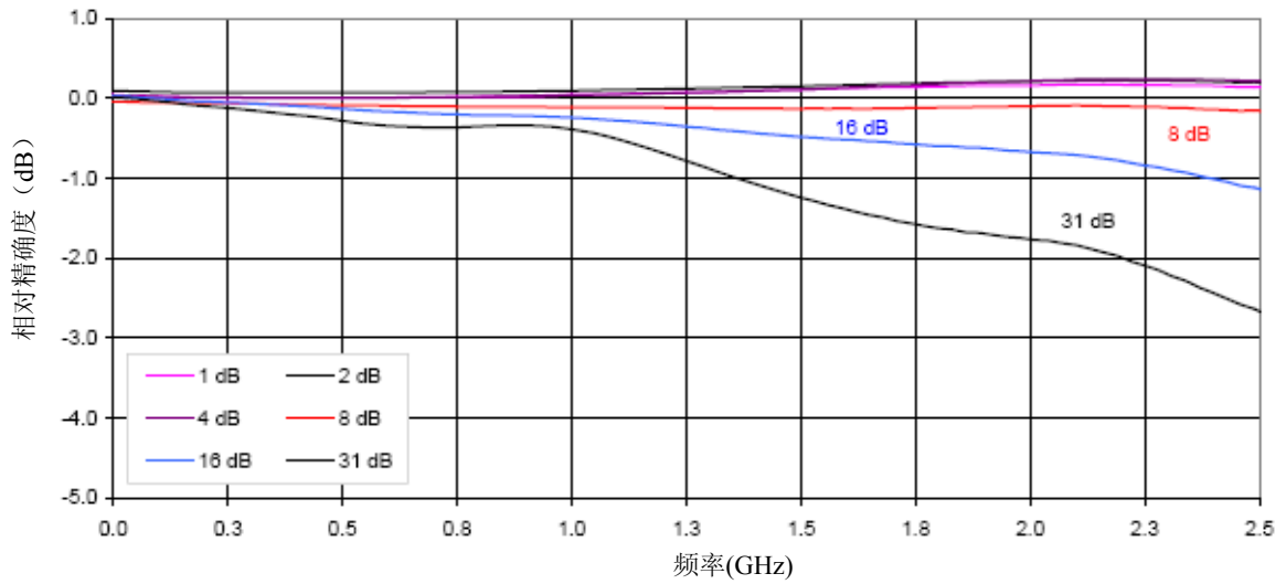
典型 AT4521 相对精度
