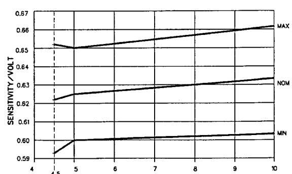
灵敏度 / V VS V_s
