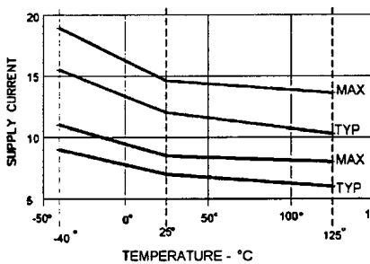
供电电流 VS 温度
