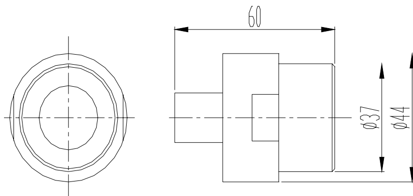
图 1: 传感结构尺寸
