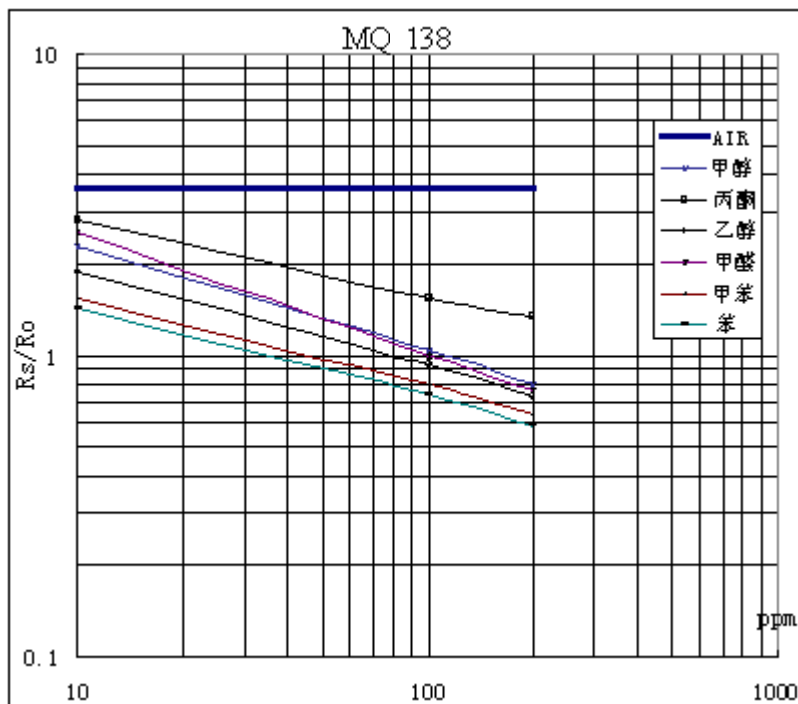
图 3 MQ138灵敏度特性曲线
