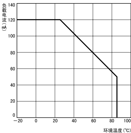
负载电流 - 环境温度 G3VM-2(F)L
