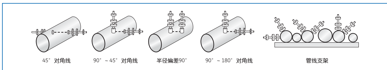
标准的火炬气流量计安装方式
