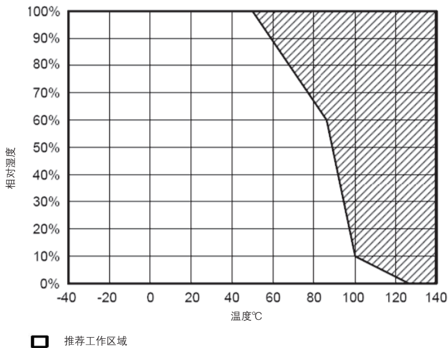
图 2. 储存环境 (仅用于非冷凝环境)
