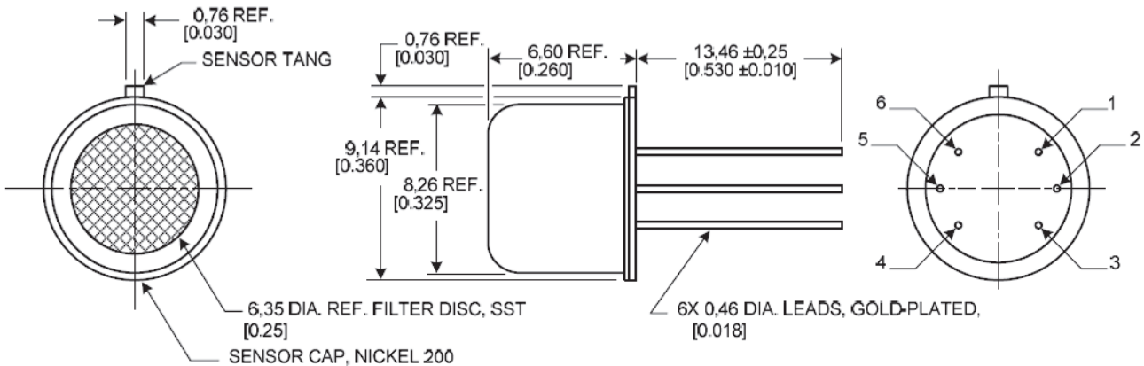
图 5.HIH-4602-A/C 系列安装尺寸 (仅供参考。mm[in])
