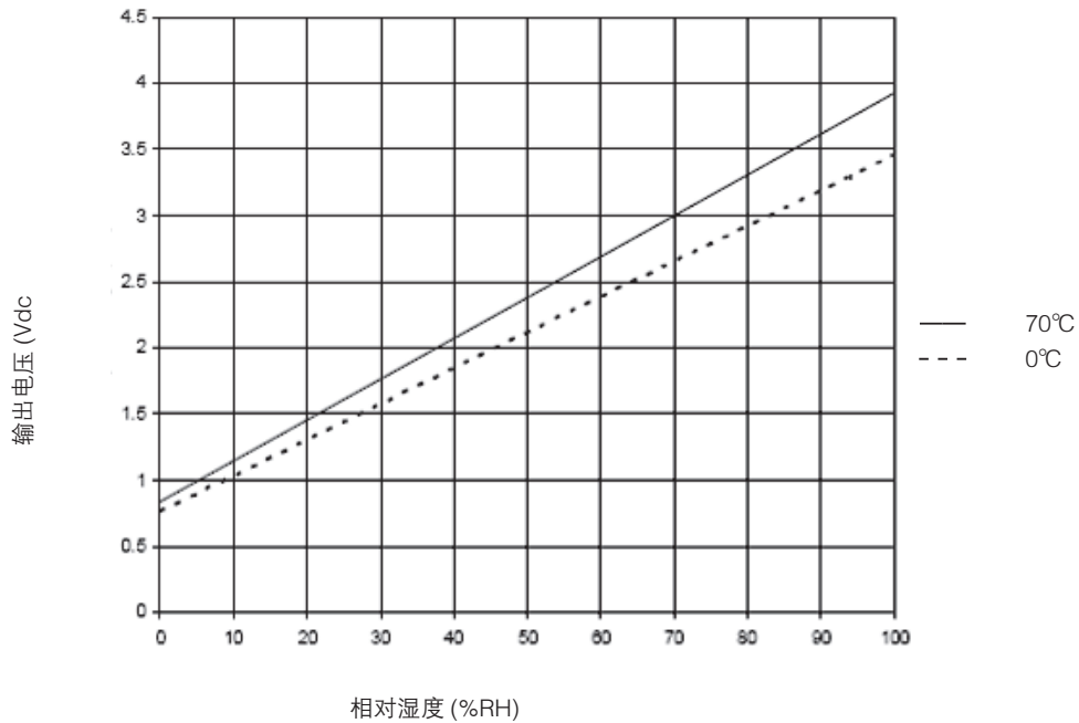
图 4. 对应相对湿度的典型输出电压 (最佳拟合直线)(在 0 °C, 70 °C 和 5V 电压下)
