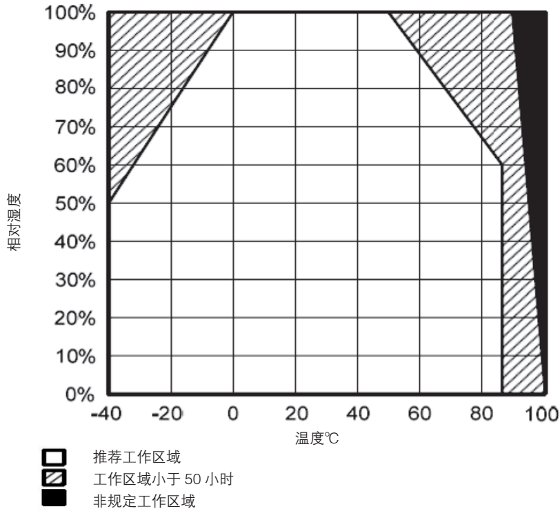
图 1. 工作环境 (仅用于非冷凝环境)
