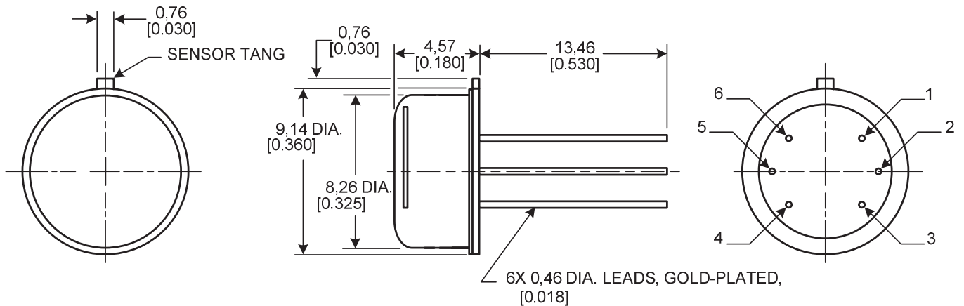
图 5.HIH-4602-L 系列安装尺寸(仅供参考。mm[in])
