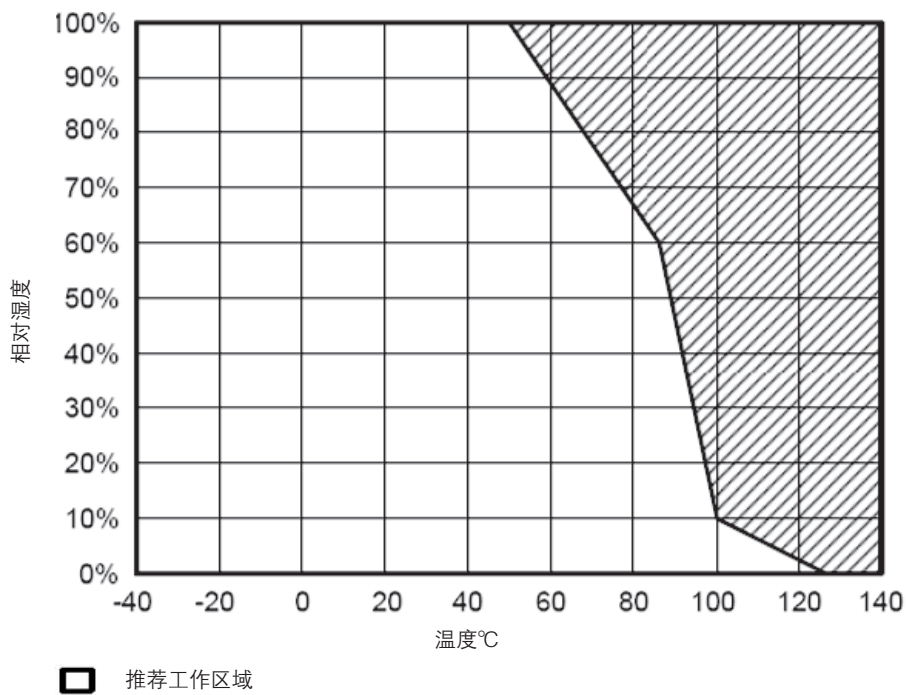
图 2. 储存环境 (仅用于非冷凝环境)
