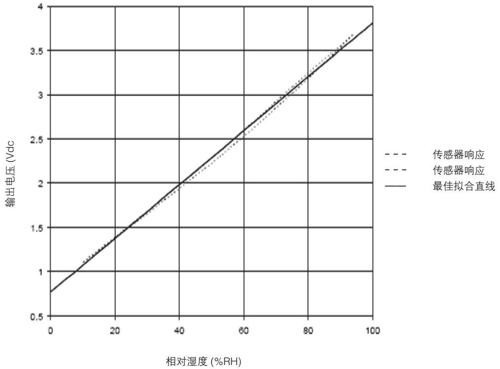
图 4. 对应相对湿度的典型输出电压 (最佳拟合直线)(在 0 °C, 70 °C 和 5V 电压下)
