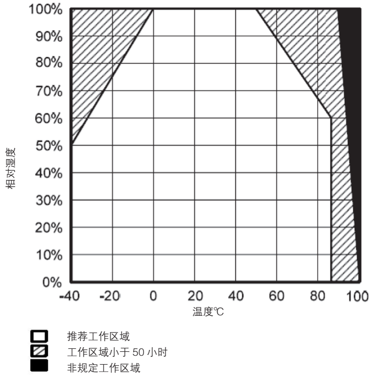
图 1. 工作环境 (仅用于非冷凝环境)
