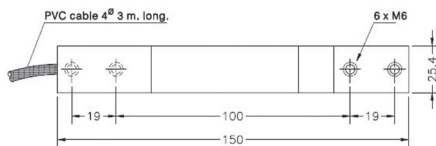
Rozměry v mm Dimensions in mm
