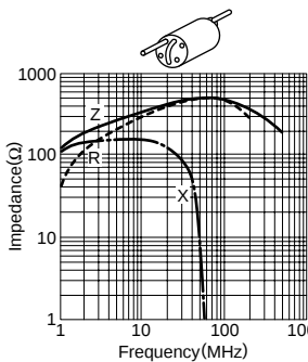
HF70R6H6X10H0.8 (3 holes)
