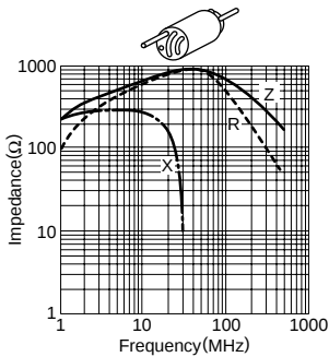
HF70R6H6X10H0.8 (5 holes)
