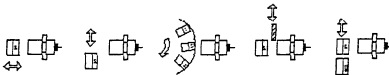
a) 轴向接近 b) 径向接近 c) 旋转 d) 遮断 e) 自锁
