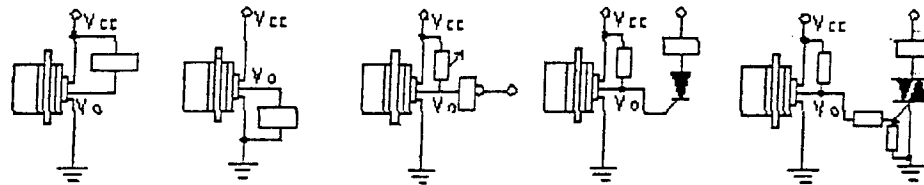
a) NPN 输出 同负载连 b) PNP 输出 同负载连 c) NPN 型同数 字电路连接 d) NPN 型同单向 可控硅连接 e) NPN 型同双向 可控硅连
