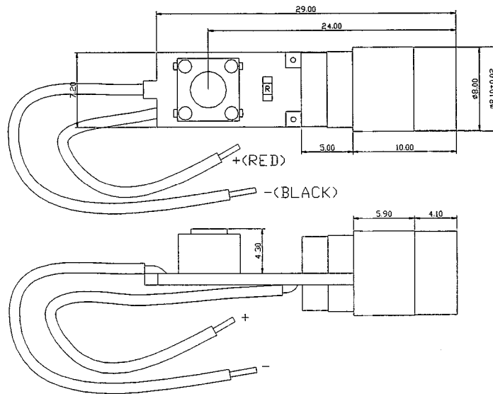
2-LMS29B-3L Supply Voltage : 3V Output Power : 2.5~5mW Iop : 25mA
