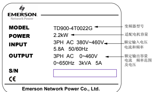
图2-1 变频器铭牌
