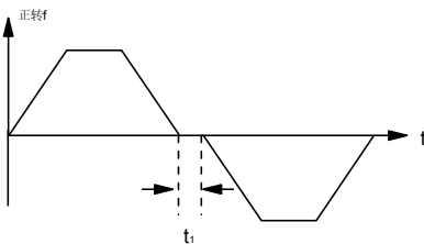
图6-5 正反转死区时间
