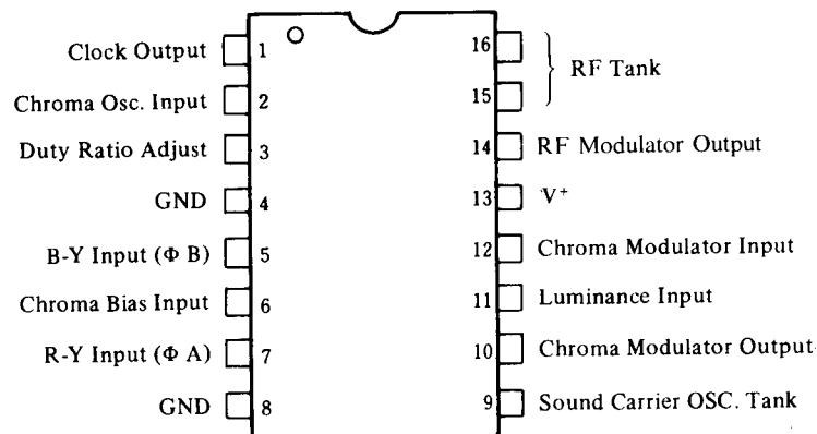
NJM2208D
