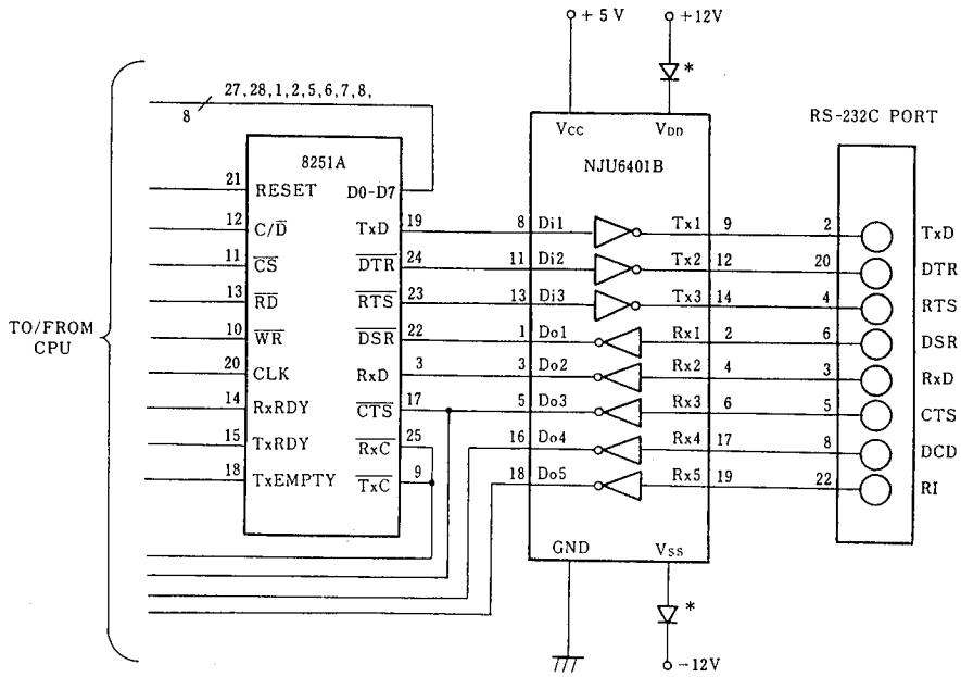
RS-232C port
