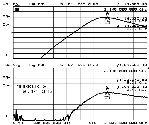
S21, S12
